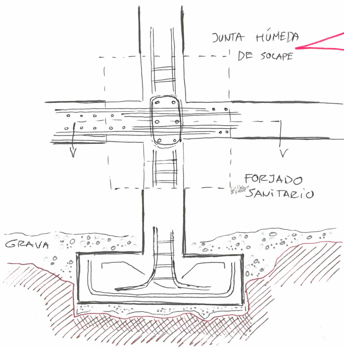
SECCIÓN DE FORJADO POR ESTRUCTURA PRINCIPAL PILAR-VIGA
