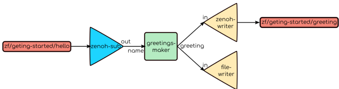
Figura 4.2: Flujo de datos de ejemplo en Zenoh-Flow
