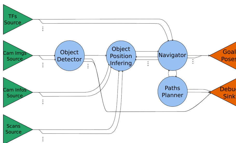
Figura 5.1: Flujo de datos de la primera versión de swarm_obj_finder
