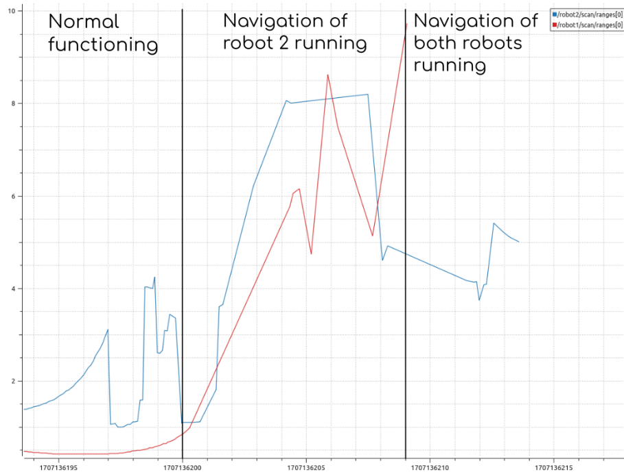
Figura 5.5: Comparación de mensajes variando la cantidad de robots
