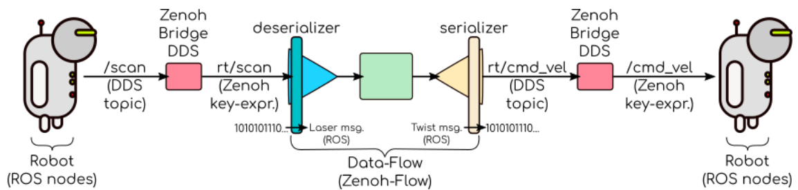
Figura 4.3: Topología software con ROS (DDS) y Zenoh-Flow (Zenoh)
