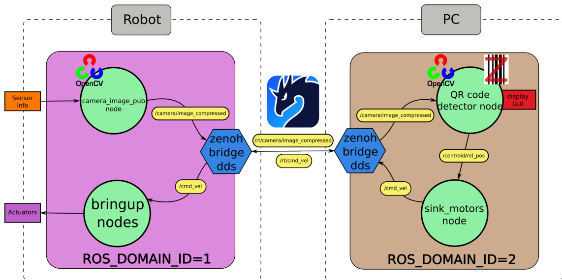
Figura 1.9: Flujo de datos de un robot para seguir códigos QR
