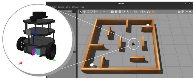
Figura 3.7: Simulación en Gazebo del Turtlebot 3 en un mundo virtual [Yuhong, 2022]
