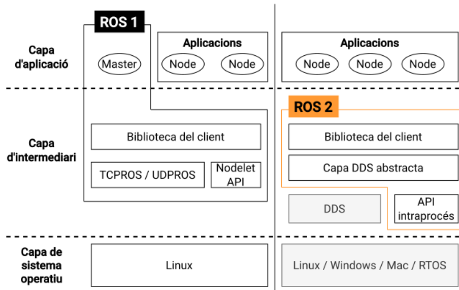
Figura 1.6: Arquitecturas de ROS y ROS2 [Auledas, 2024]
