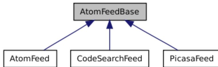
Figura 3.5.3: Diagrama de herencia de la clase AtomFeedBase
