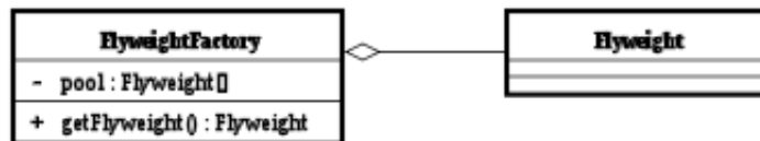
Figura 3.5.5: Arquitectura del patrón Flyweight
