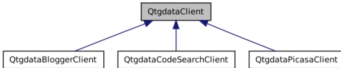
Figura 3.5.4: Diagrama de herencia de la clase QtgdataClient
