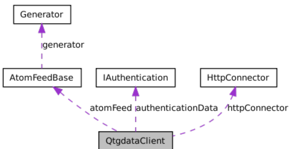
Figura 3.5.2: Diagrama de colaboración de la clase QtgdataClient
