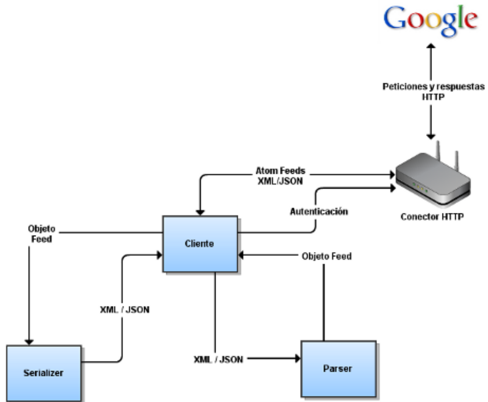
Figura 3.1.1: Arquitectura cliente-servidor de alto nivel del Protocolo de Datos de Google
