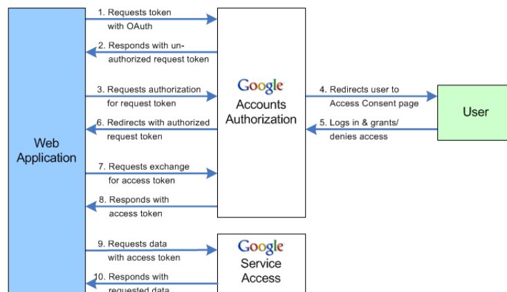
Figura C.1.1: Diagrama de flujo del proceso OAuth
