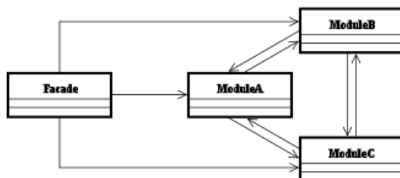
Figura 3.5.1: Estructura del patrón de diseño Facade
