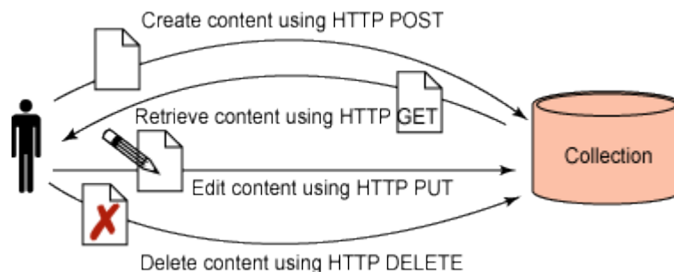
Figura B.1.1: El Protocolo Atom emplea simples peticiones HTTP para publicar y modificar contenido
